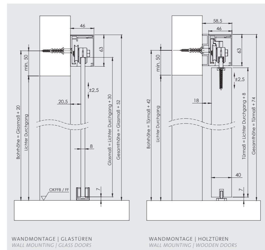
PLANE0 60 PRO VOR DER ZARGE IN FRONT OF FRAME
